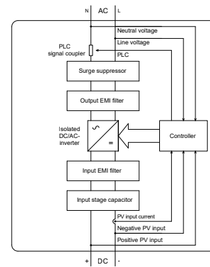
IQ9N Microinverter
