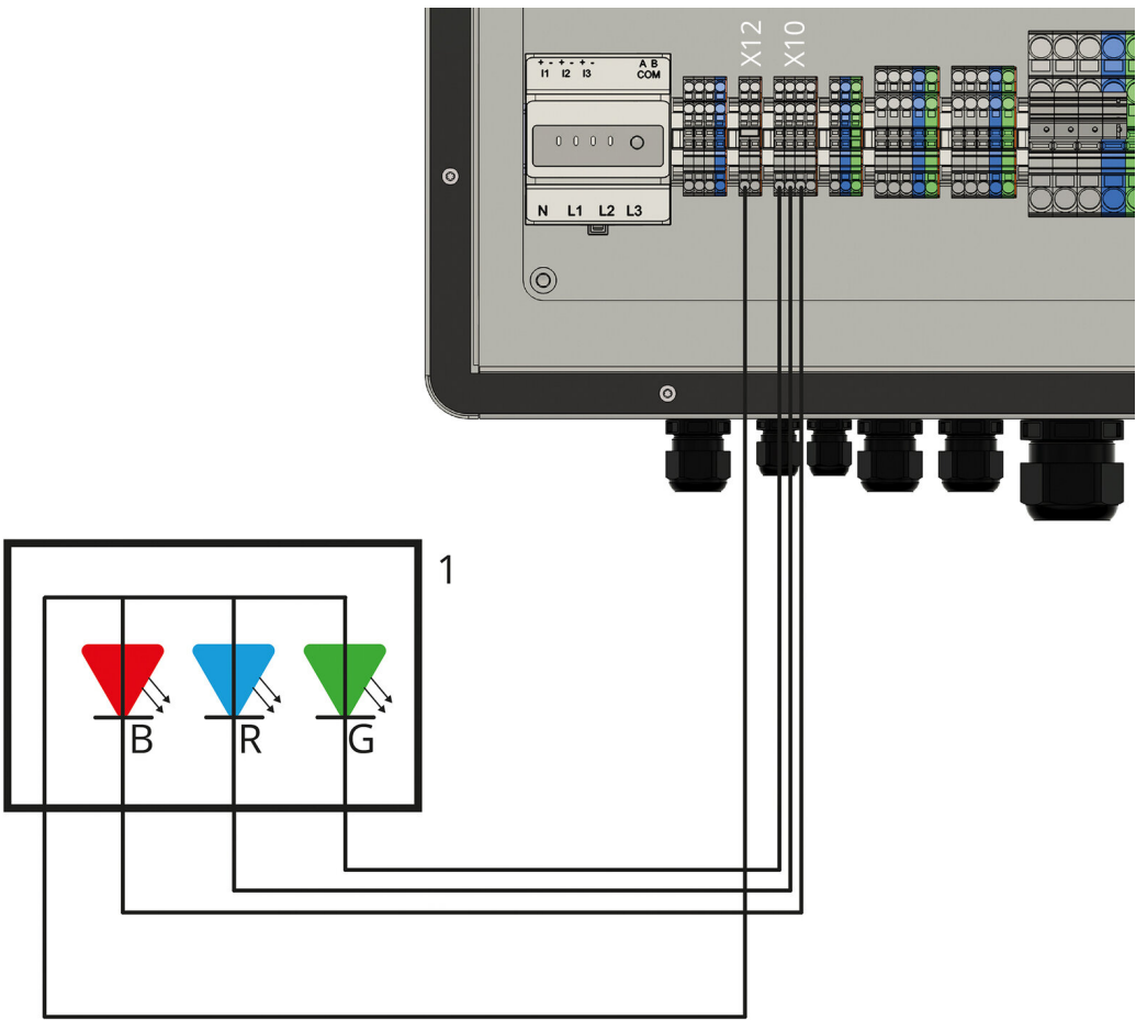
Abbildung 10. Anschluss externe Statusanzeige
