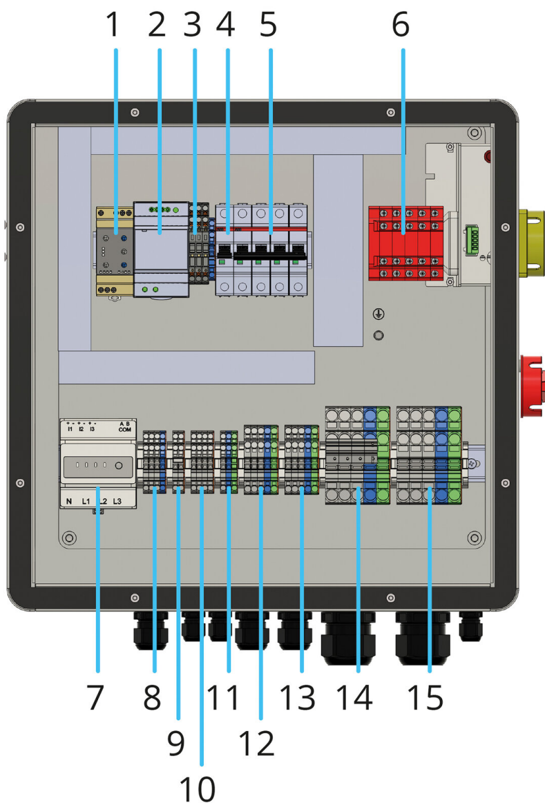
Abbildung 2. Übersicht — Innenaufbau — AVU
