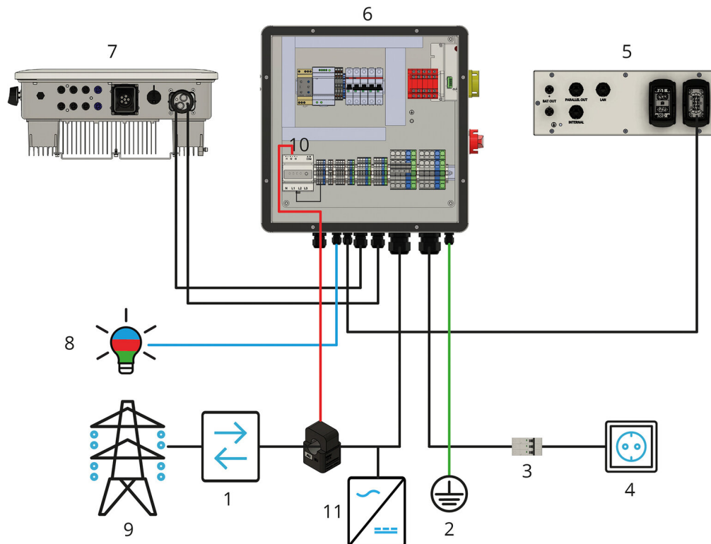
Abbildung 11. Installationsübersicht mit externem AC-Erzeuger
