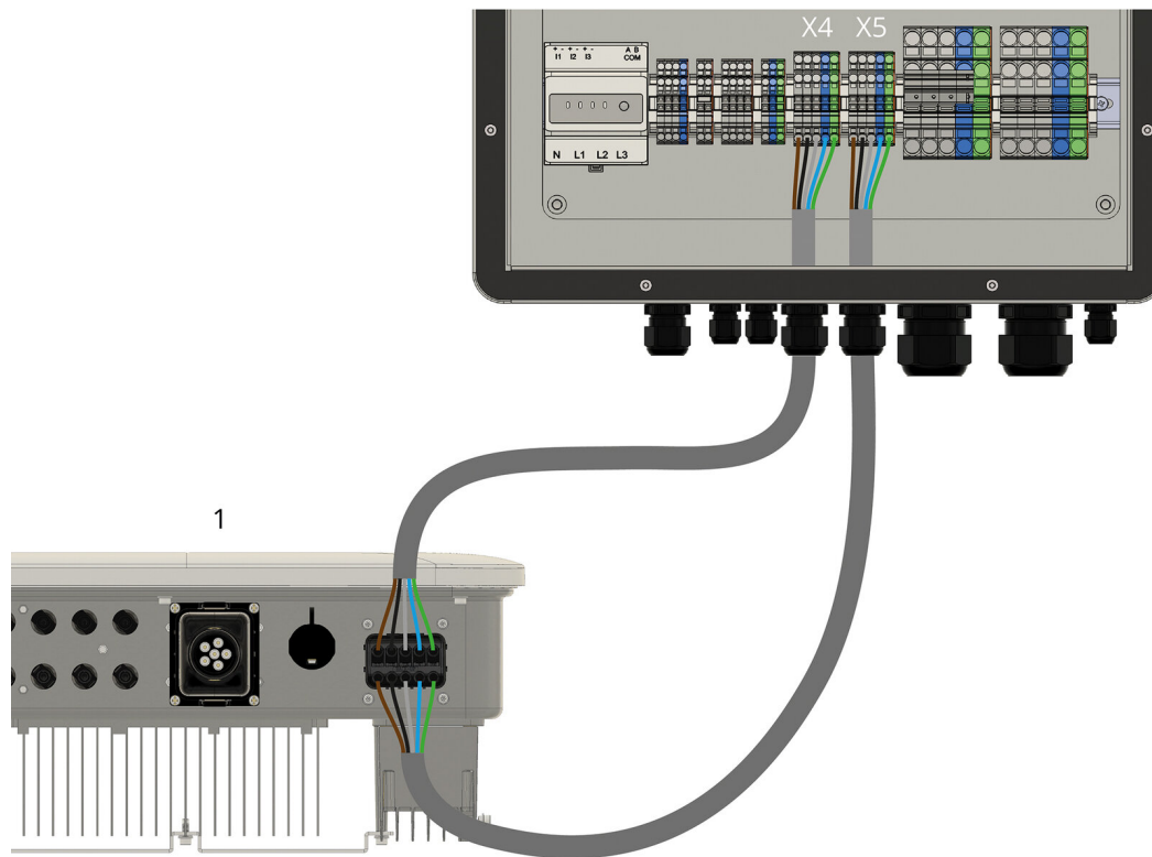
Abbildung 7. AC-Anschluss — Wechselrichter
