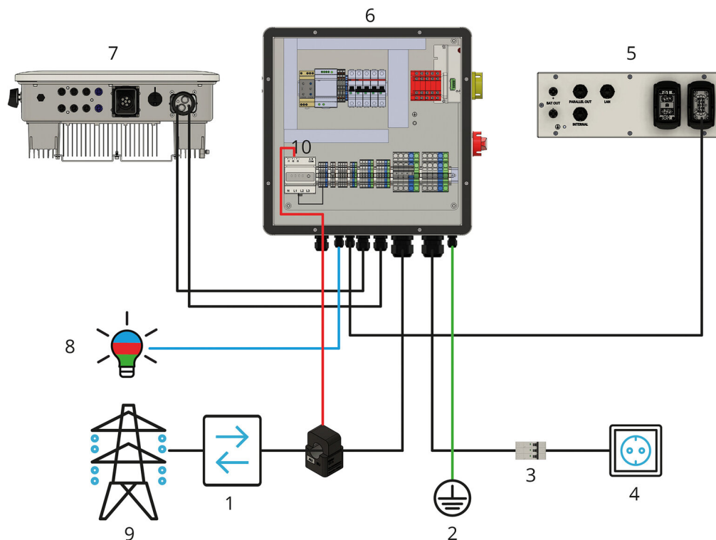
Abbildung 6. Gesamtübersicht der Anschlussverbindungen
