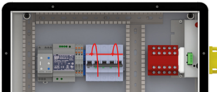
Abbildung 16. Einsichern der Leitungsschutzschalter in der AVU
